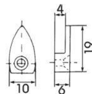
Taquet pour fixation de miroir en plastique
